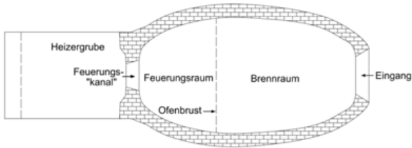
1 Prinzip eines Freifeuer-Keramikbrennofens. Grundlage für diese Rekonstruktionsvorlage ist ein Steinzeug-Brennofenbefund in Frechen, Hauptstraße 3-7 (Periode 1) (S. Döbel nach Vorlage durch den Autor).
