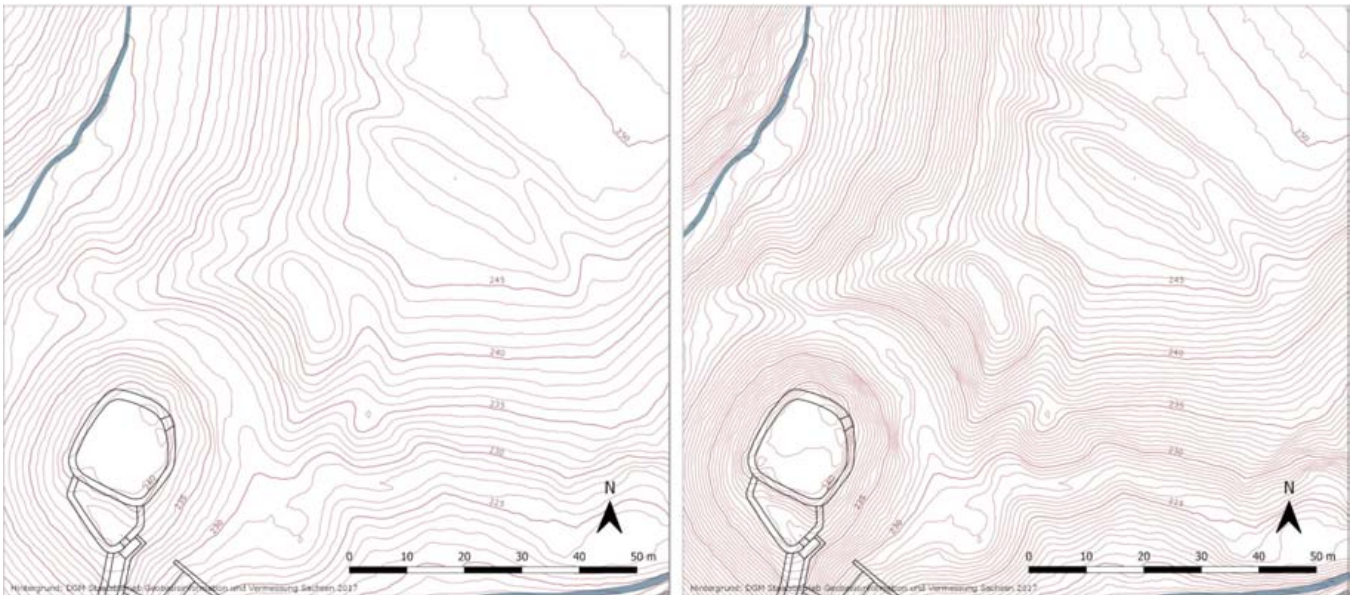
3 Detailausschnitt des nordöstlichen Bereichs der Burg Helfenberg. Im Vergleich zwei Höhenlinienpläne mit Höhenlinienabständen von 1,0 Meter (links) und 0,5 Meter (rechts) (Geländemodell aus Daten des Staatsbetriebs Geobasisinformation und Vermessung Sachsen, 2017).
